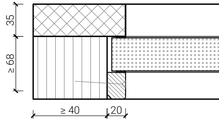
Glas bündig RC4 / FB4-Doppel
