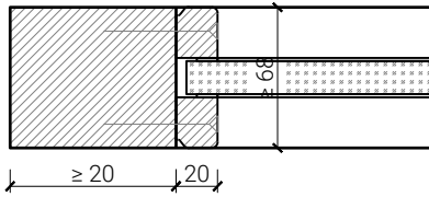
Glas / Füllung mittig Glasleiste einseitig
