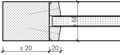
Glas / Füllung mittig Glasleisten Gerade
